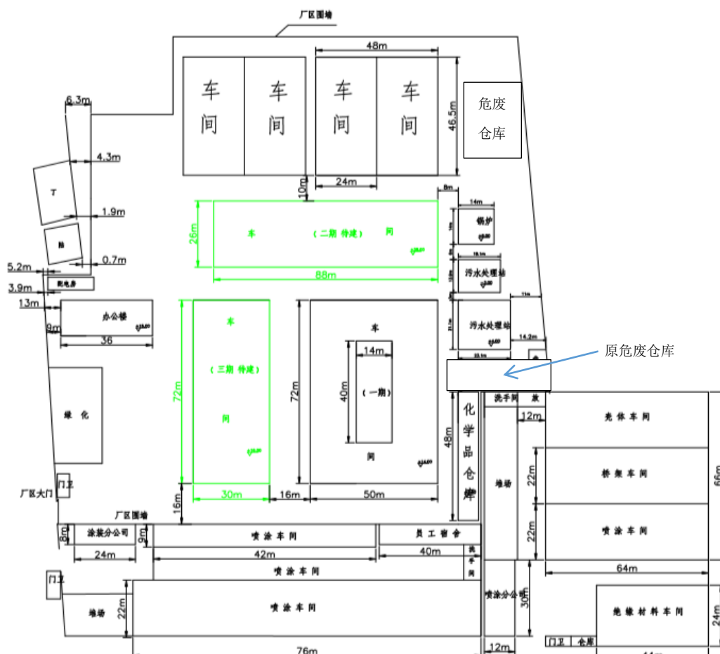
图 3-7 宏飞镀业平面布置图
