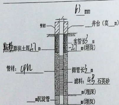
井结构示意图
