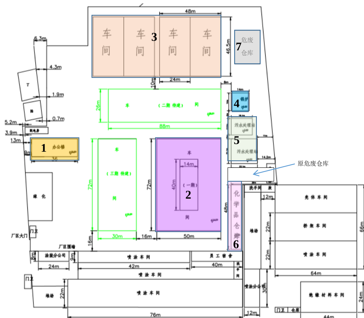
图 4-2 企业平面布置中重点区域划分情况图
