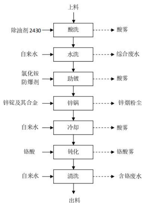
图 4-2 热镀锌生产工艺流程图
