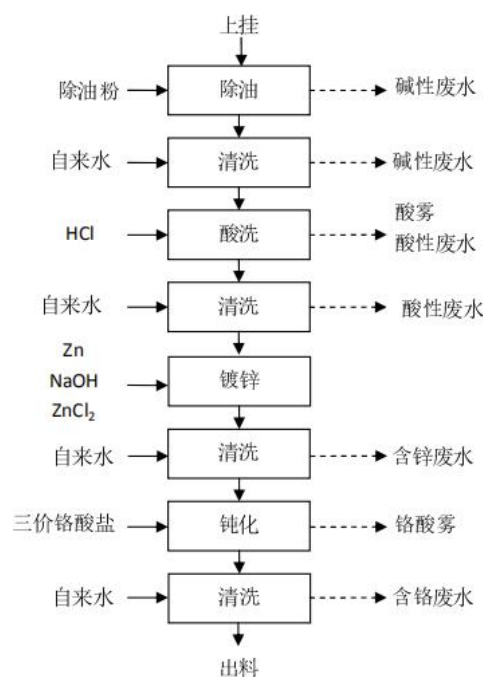
图 4-3 镀锌生产工艺流程图
