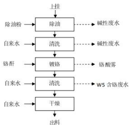
图 4-5 镀铬生产工艺流程图
