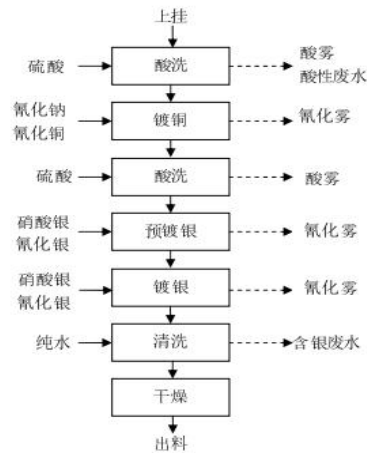
图 4-6 镀银生产工艺流程图
