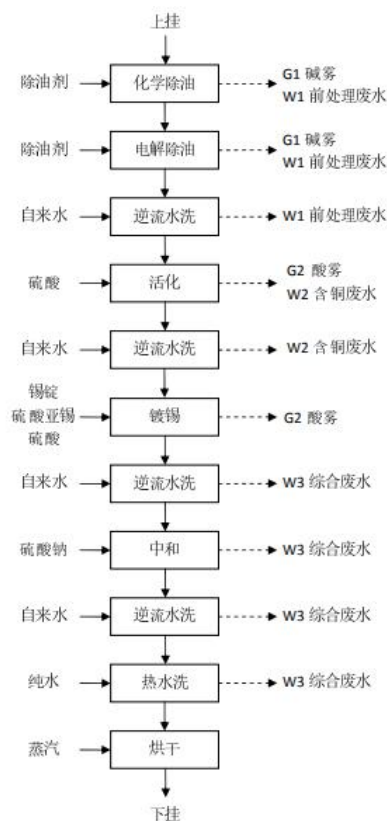
图 4-1 铜排镀锡生产工艺流程图
