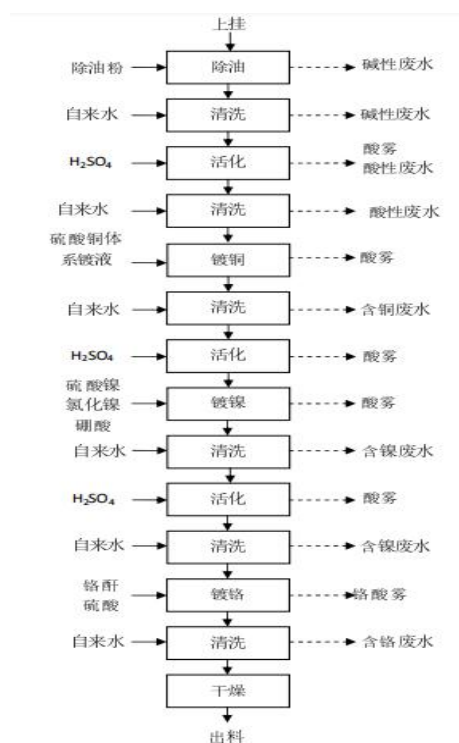
图 4-4 镀镍生产工艺流程图
