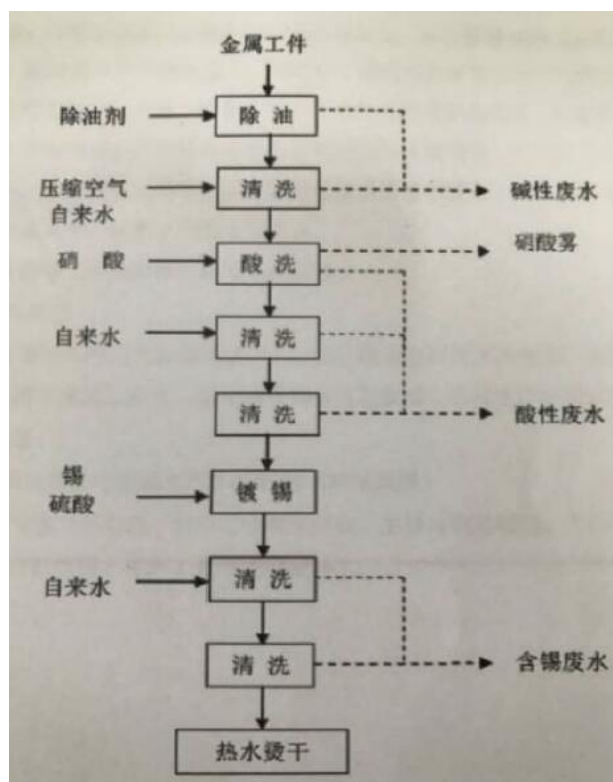
图 4-4 镀锡生产工艺流程图
