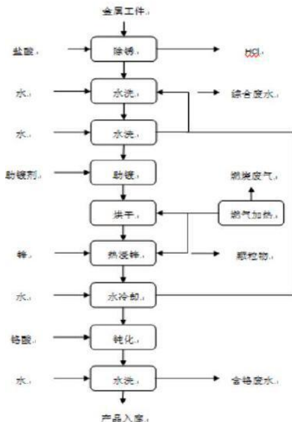
图 4-1 热浸锌生产工艺流程图
