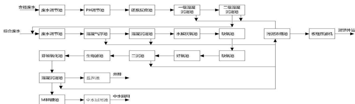
图 4-5 污水处理工艺流程图
