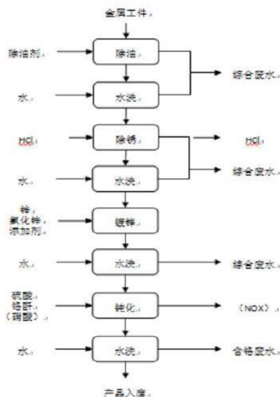
图 4-2 镀锌生产工艺流程图
