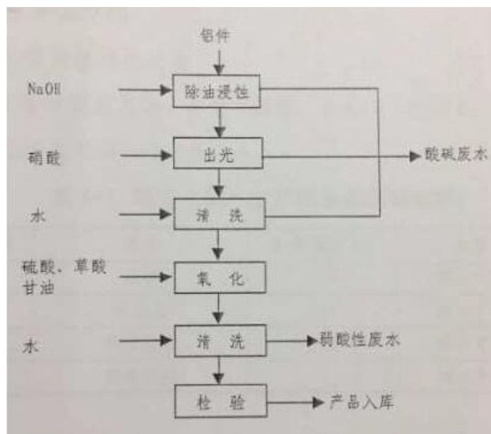
图 4-3 铝氧化生产工艺流程图
