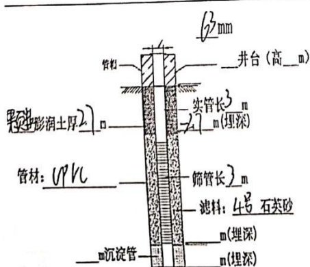
井结构示意图
