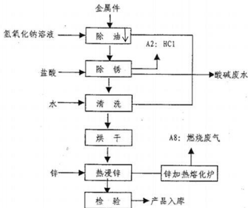
图 4.1.1-1 热浸锌生产工艺流程图
