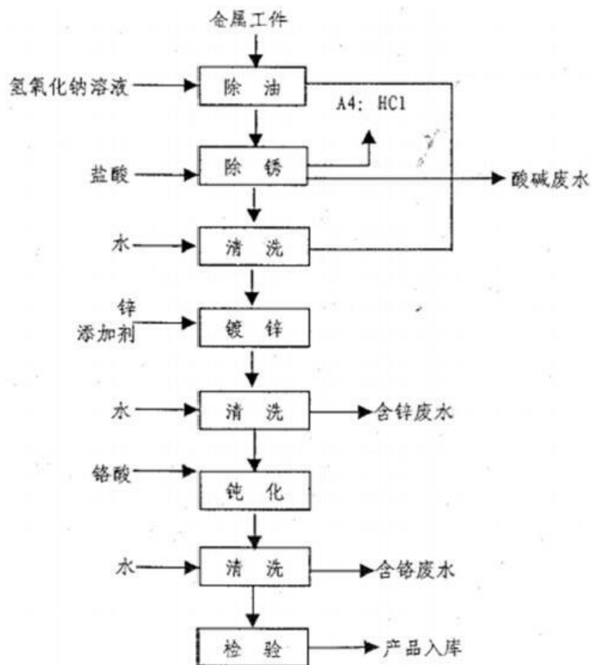
图 4.1.1-2 镀锌生产工艺流程图
