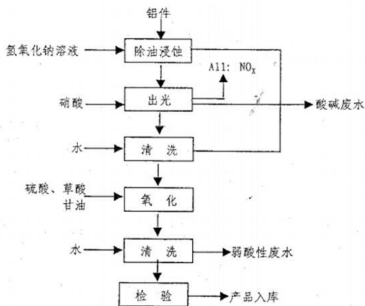
图 4.1.1-4 铝氧化生产工艺流程图
