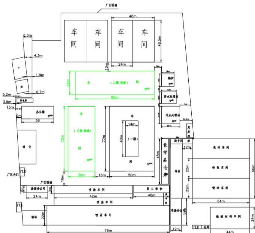
图 4.2-1 企业总平面布置图
