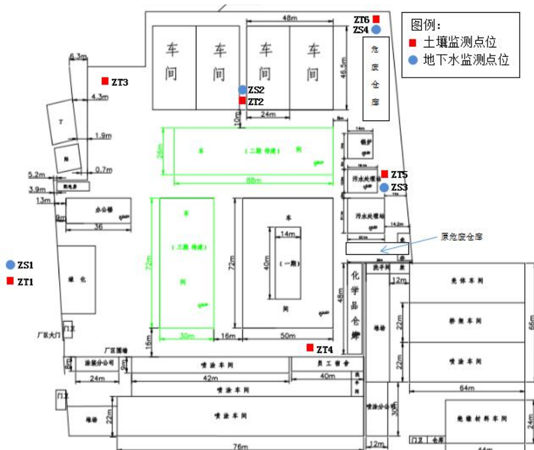
图 6-2 监测点位平面布置图
